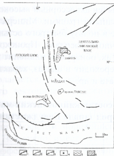
Рис.1. Тектоническая схема региона. Разрывные нарушения (1-3): 1- с надвиговой компонентой; 2- достоверные; 3- предполагаемые; 4- каинзойские магматические структуры с вулканами центрального типа; 5- дно впадины в пустыне (плайя); 5- район дополнительных работ.
